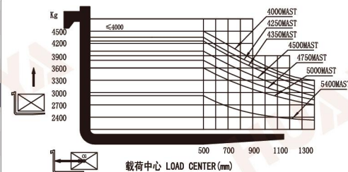
4.5T载荷曲线图 4.5T load curve
